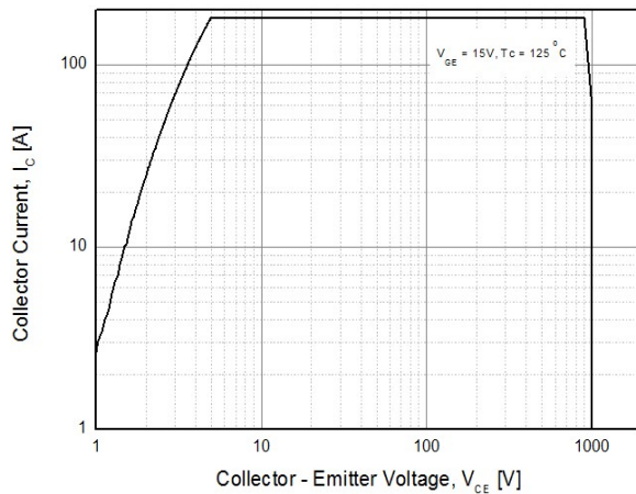
Fig. 15 RBSOA
